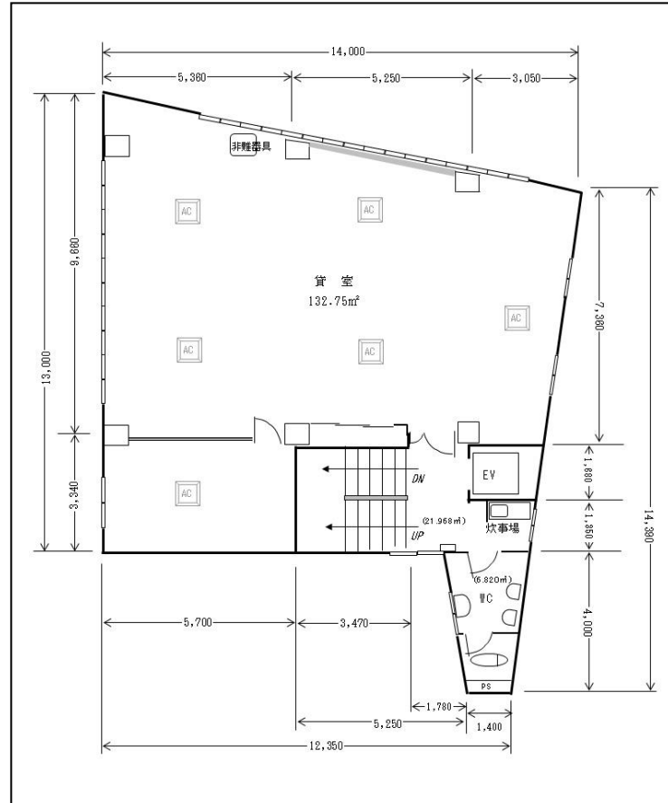
7階平面図
